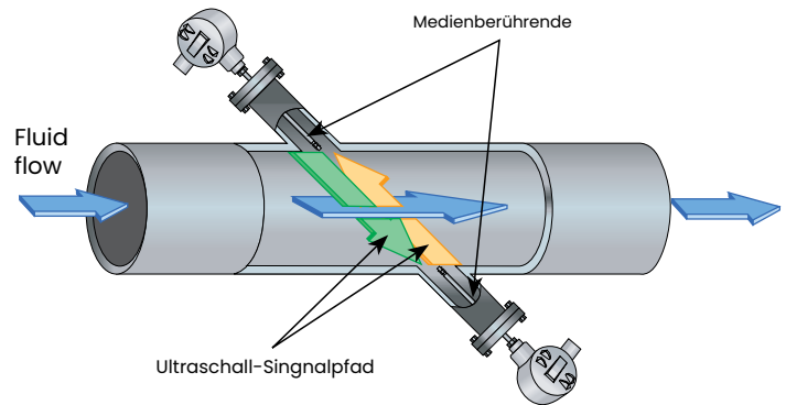
Laufzeit-Differenz-Durchflussmessungstechnik
