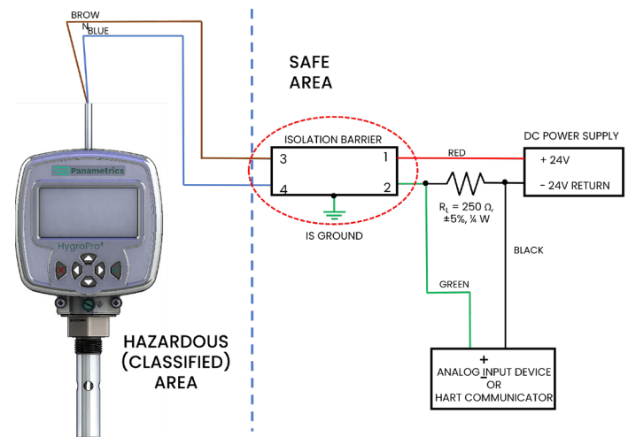
Typische Installation in explosionsgefährdeten Bereichen mit Verbindung zu einem analogen Ausgangsgerät/HART-Master mit einer optionalen widerstandsbeschränkten Isolationsbarriere
