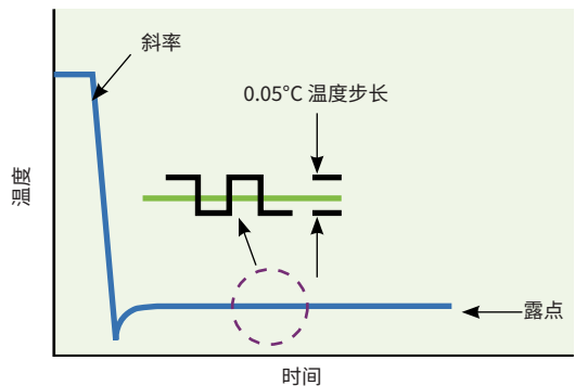
Digiloop 控制
