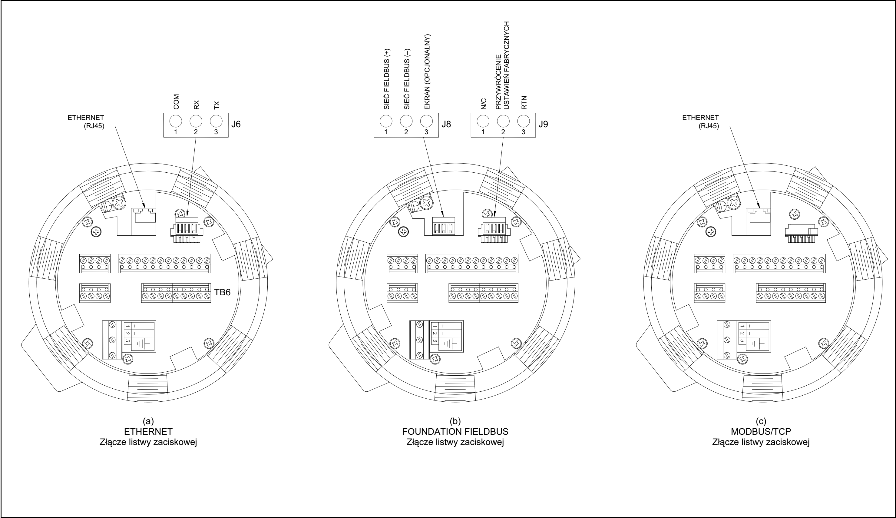
Rysunek 11: Podłączenia do listwy zacisków – Ethernet, Foundation Fieldbus oraz MODBUS/TCP
