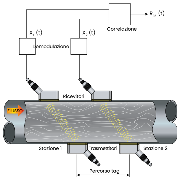
Rappresentazione schematica di un'installazione di flussimetro a Correlation Tag
