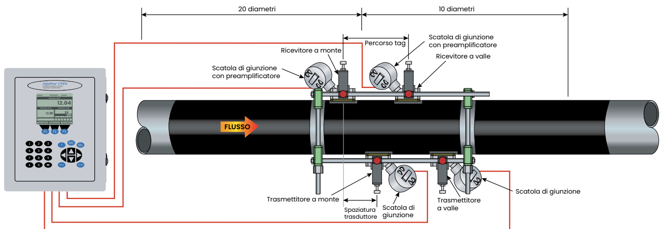
Fissaggio clamp-on V8 del DigitalFlow CTF878 con rivestimento per attenuazione del rumore
