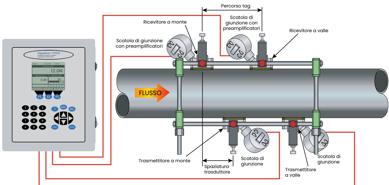
Impostazione tipica del misuratore
