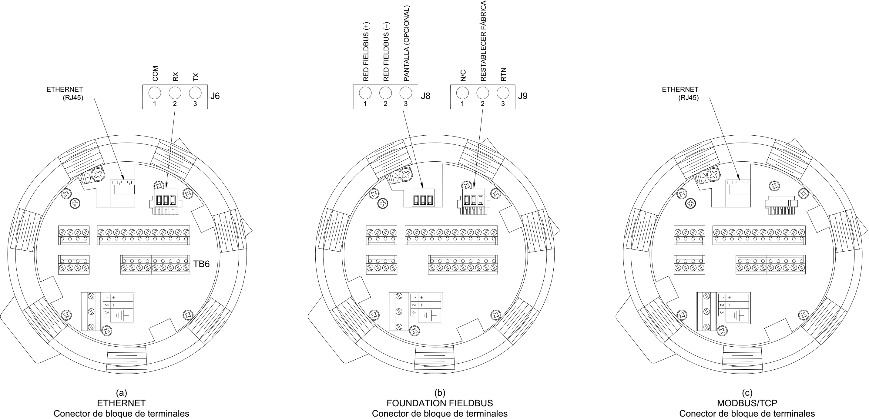
Figura 11: Conexiones del bloque de terminales - Ethernet, Foundation Fieldbus y MODBUS/TCP
