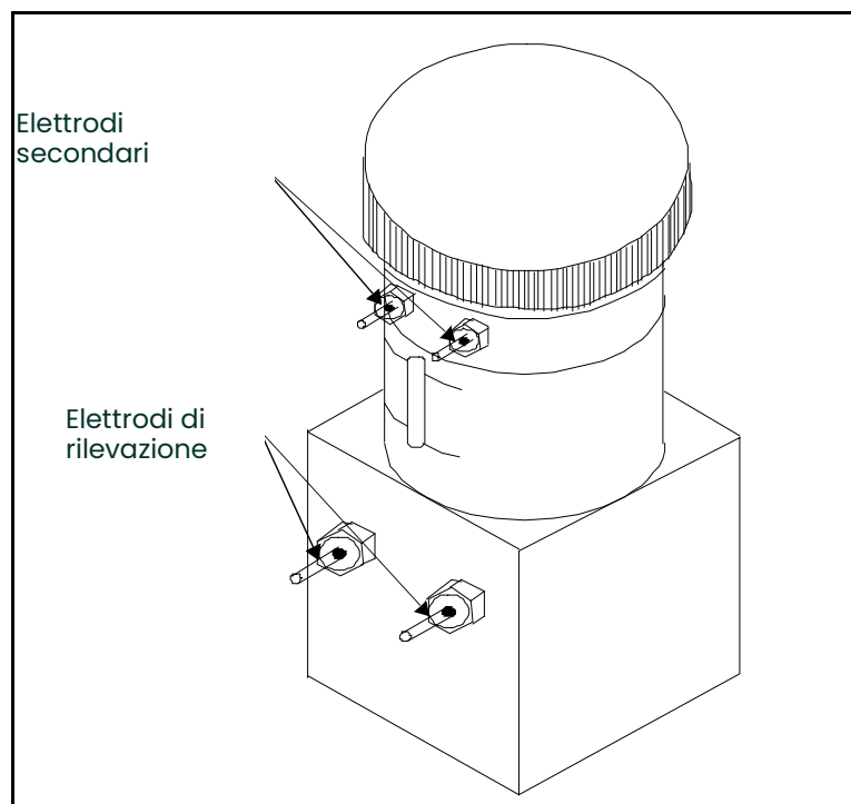
Figura 20: Cella ad ossigeno Delta F standard
