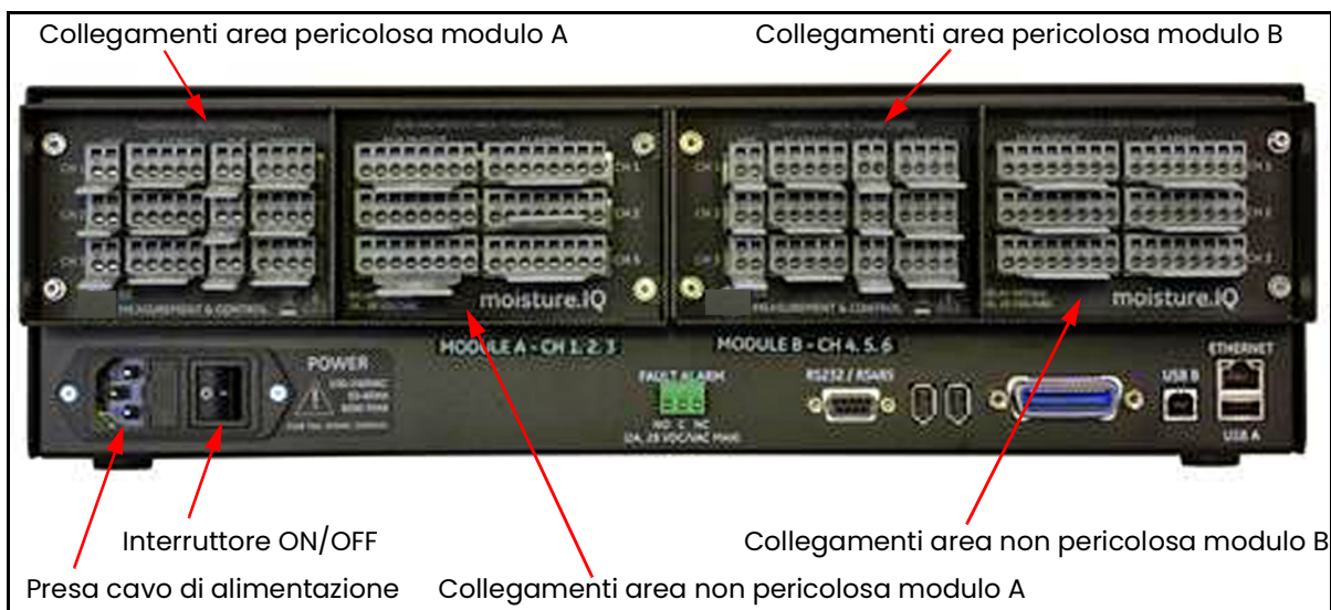
Figura 8: Collegamenti del pannello posteriore
