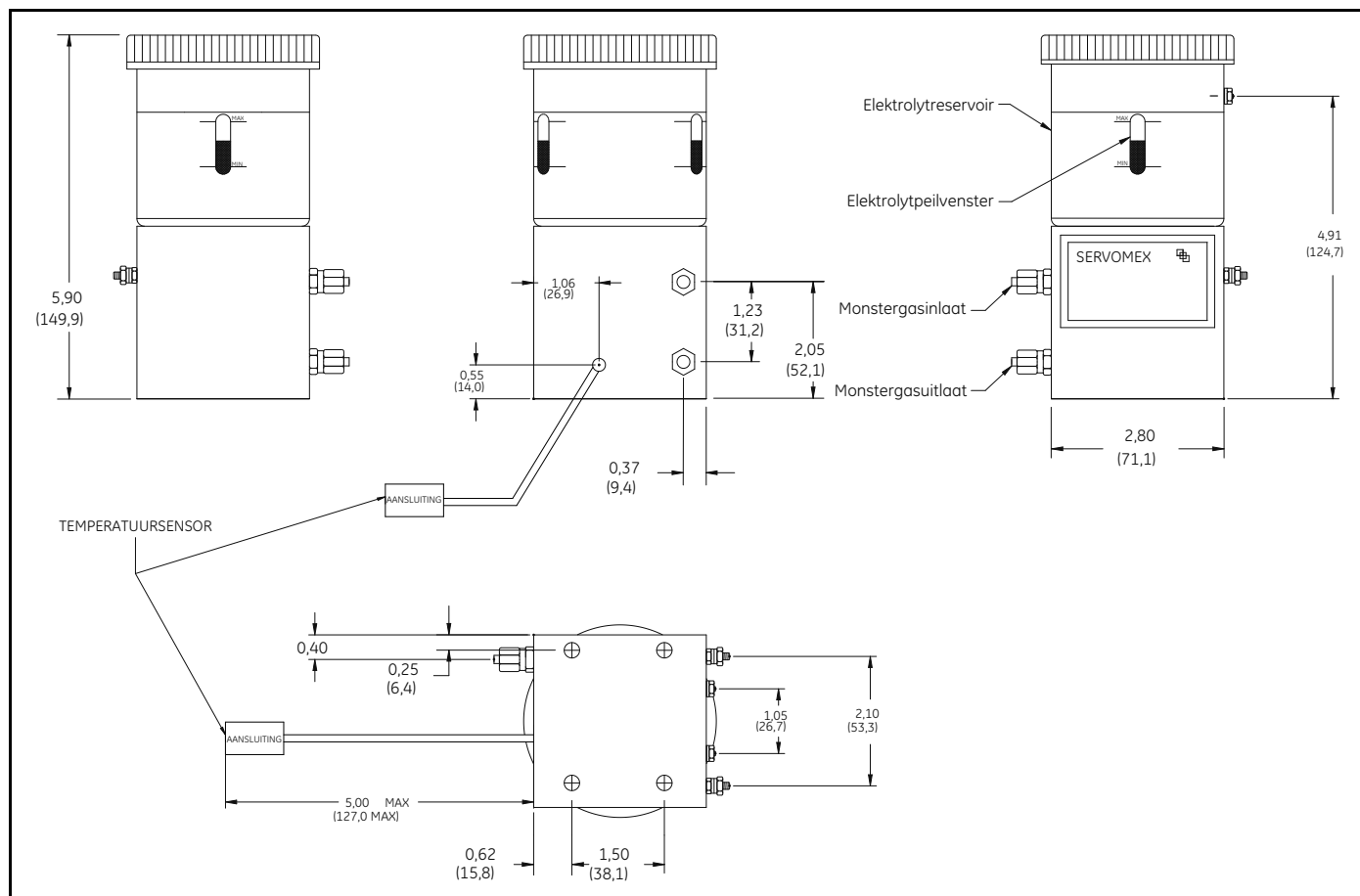
Figura 3: Dimensioni della cella ad ossigeno
