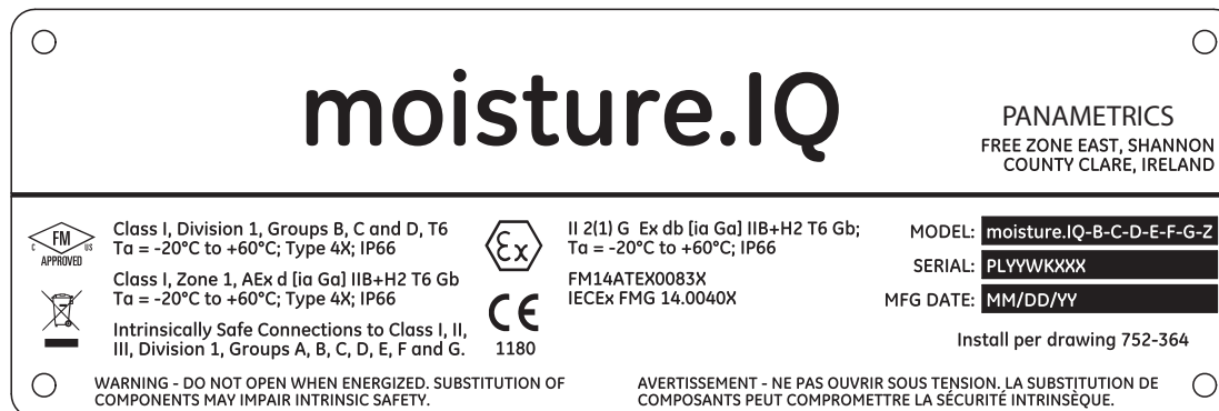
Figura 114: Etichetta a prova di esplosione da Shannon, Irlanda (Dis. 442-1855-02_revB)
