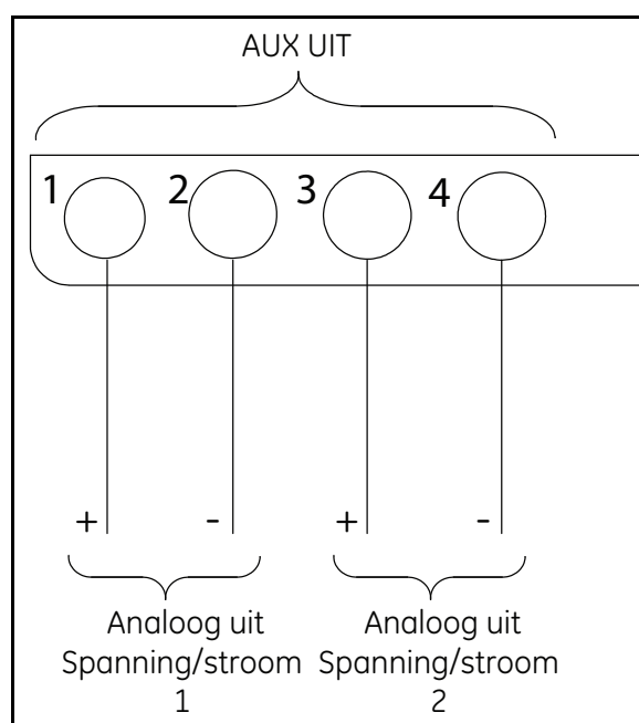
Figura 25: Cablaggio uscita
