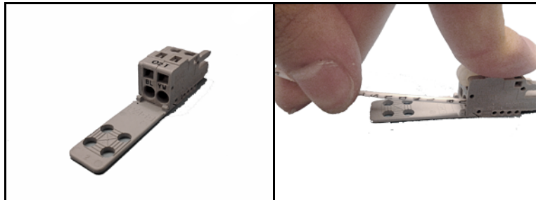
Figura 9: Utilizzo della leva di blocco a pressione
