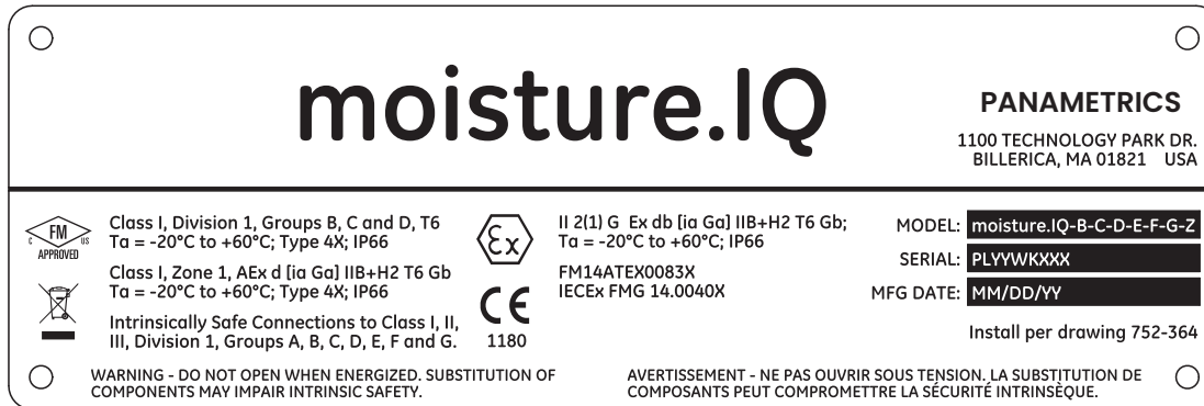
Figura 113: Etichetta a prova di esplosione da Billerica, USA (Dis. 442-1855-01_revB)
