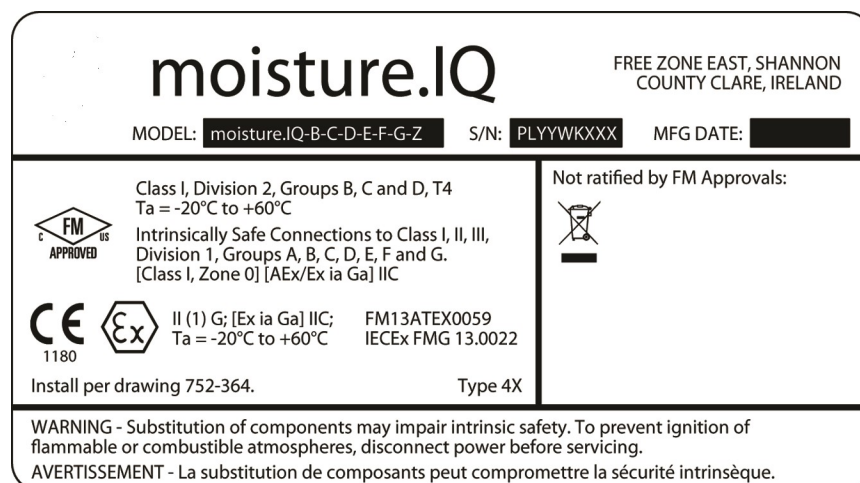
Figura 118: Etichetta impermeabile in fibra di vetro da Shannon, Irlanda (Dis. 442-1875-04_revB)
