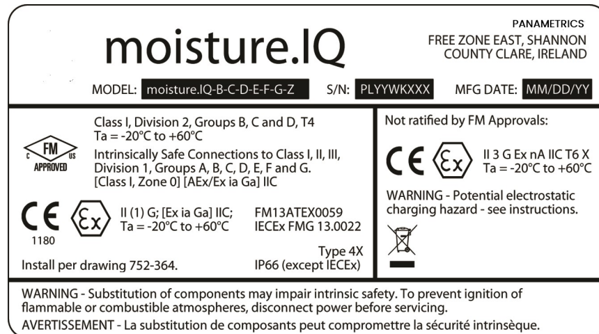
Figura 116: Etichetta impermeabile in acciaio inox da Shannon, Irlanda (Dis. 442-1875-02_revB)
