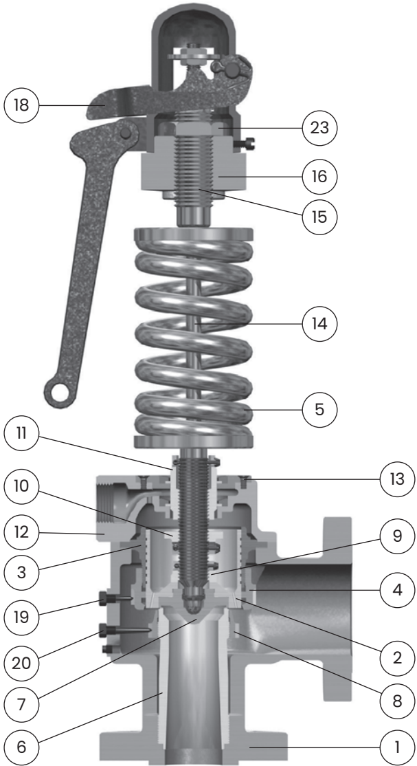
Solo números de tipo de válvula 1786-HP y 1706RR-HP
