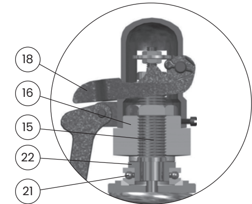
Solo números de tipo de válvula 1786-HP y 1706RR-HP
