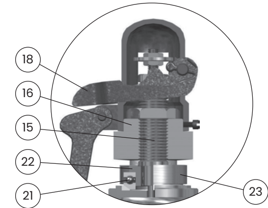
Solo números de tipo de válvula 1787 y 1707R
