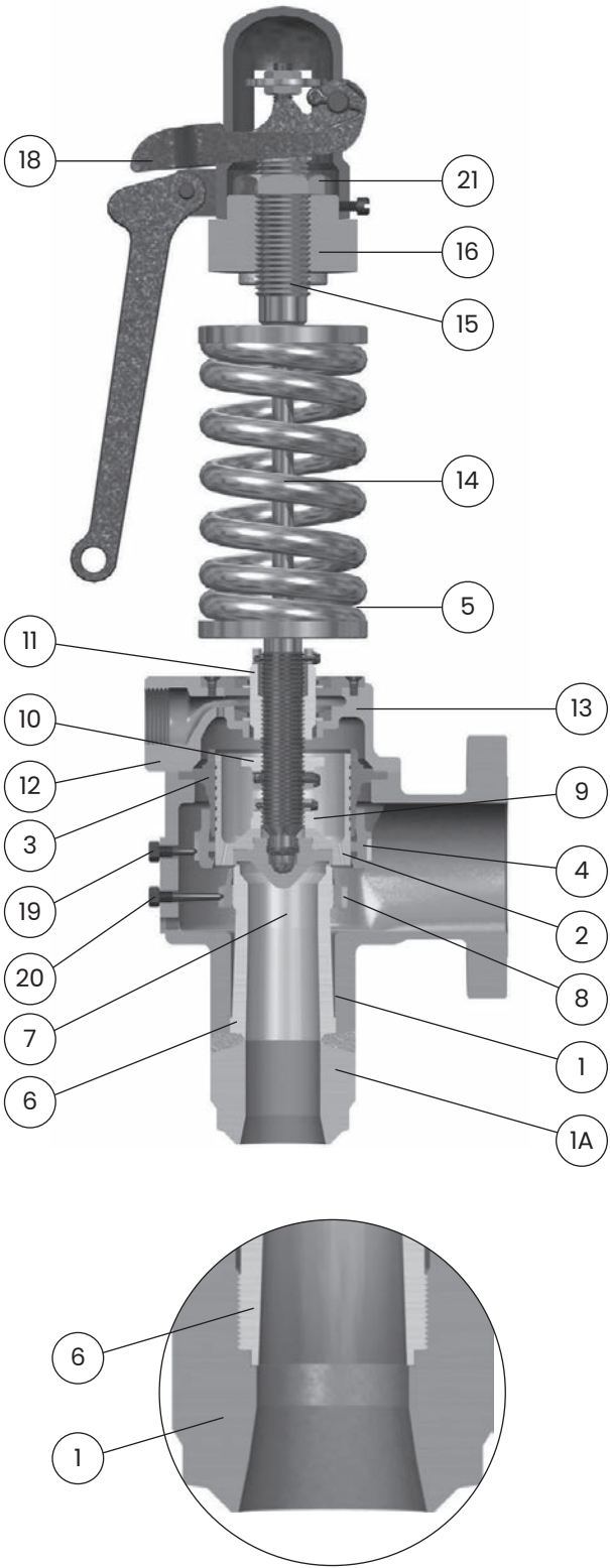
Cuello de entrada fundido de 4" a 6"
