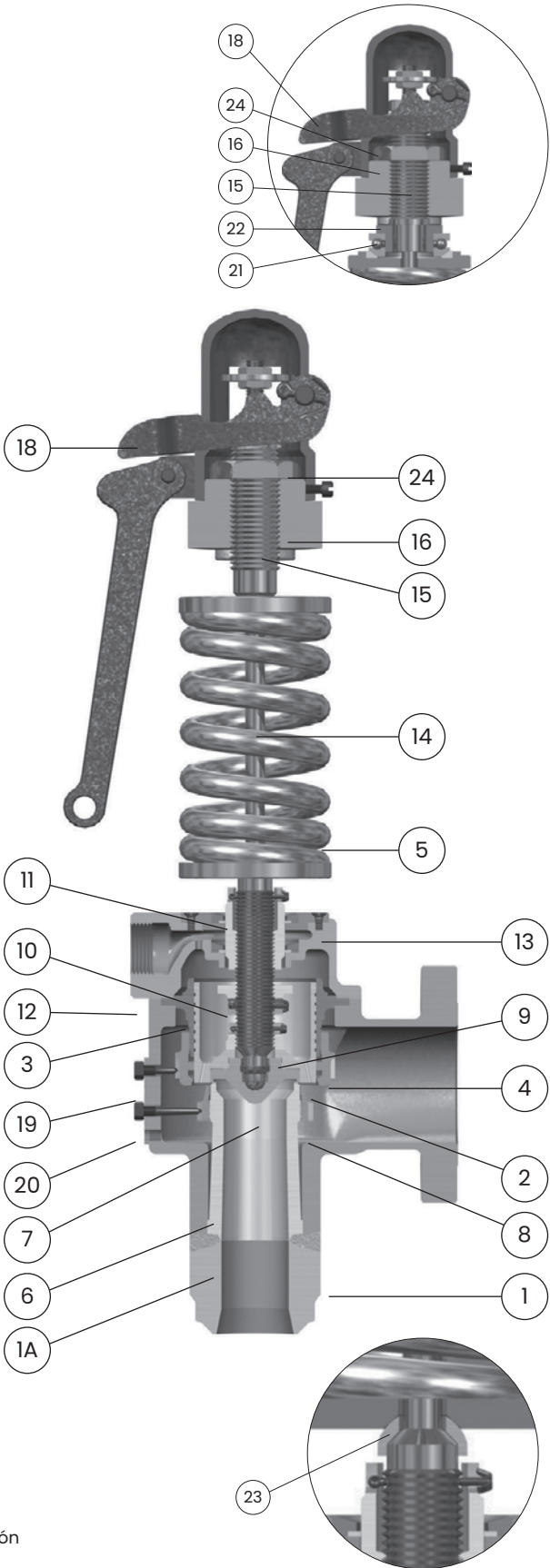
Solo número de tipo de válvula 1719
