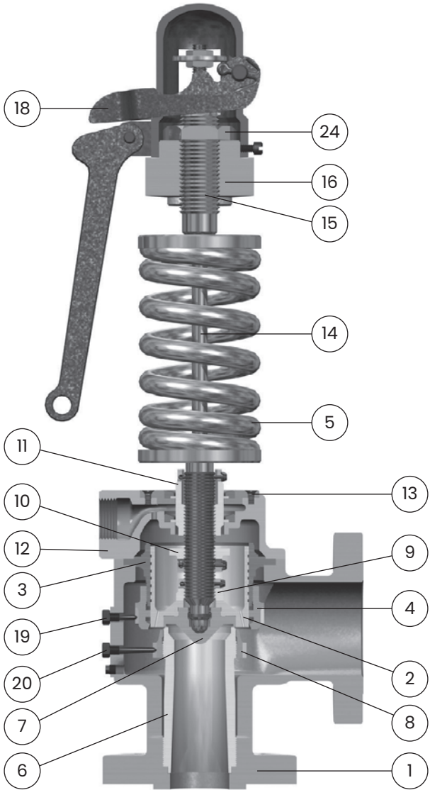
Solo números de tipo de válvula 1787 y 1707R
