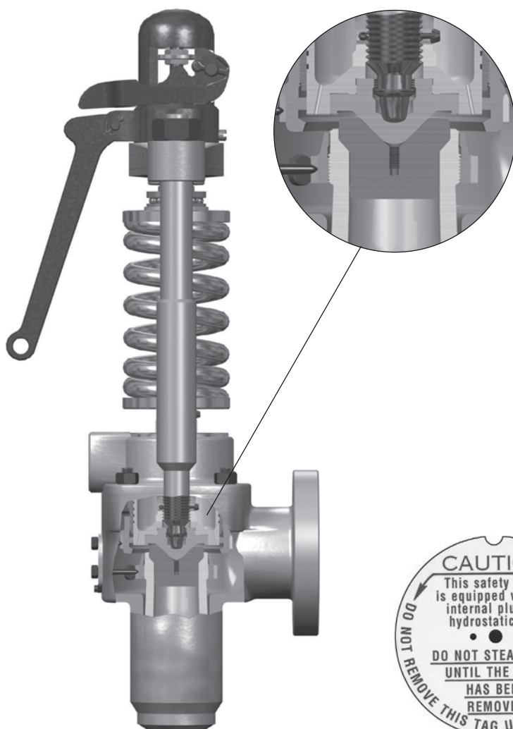
Válvula de seguridad de la serie 1700
