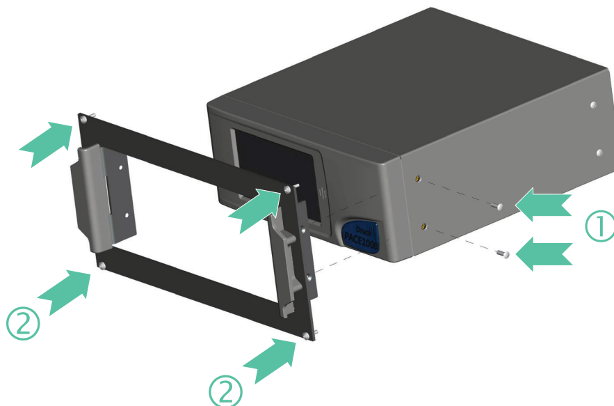
图 2-5：面板安装
