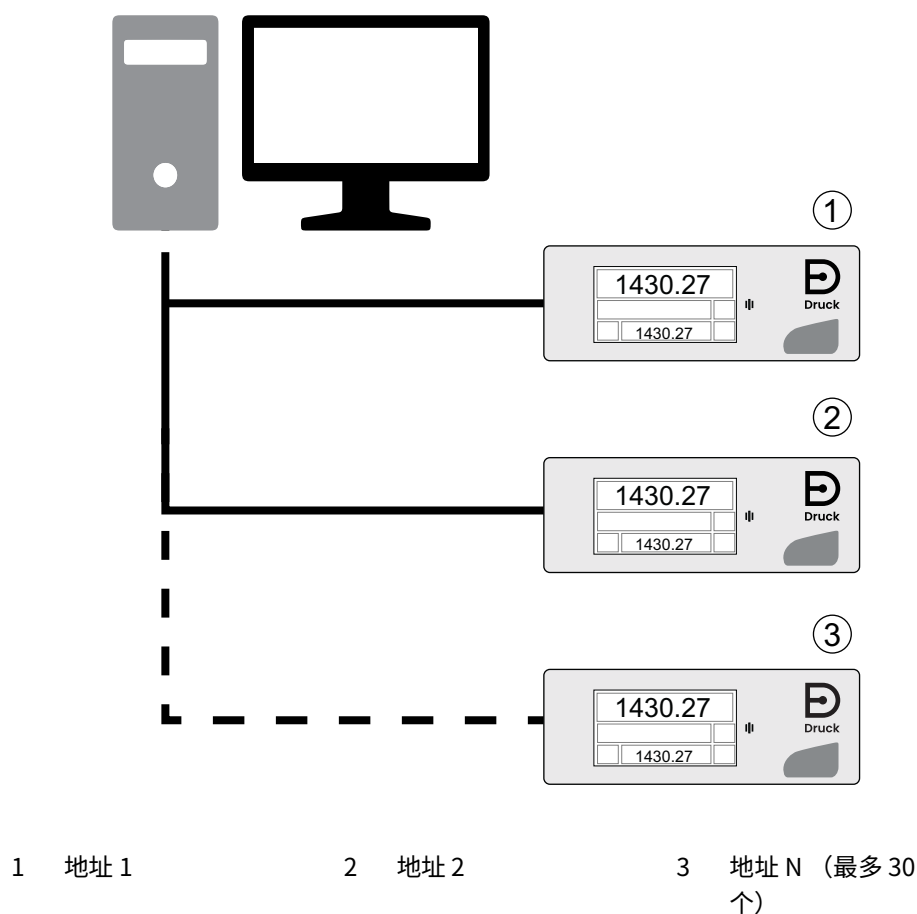
图 2-7: IEEE 488 连接
