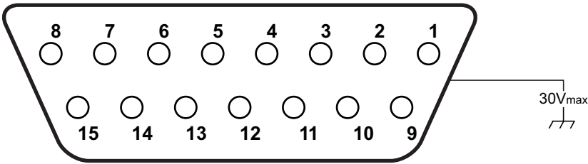
图 8-2：连接器前 View
