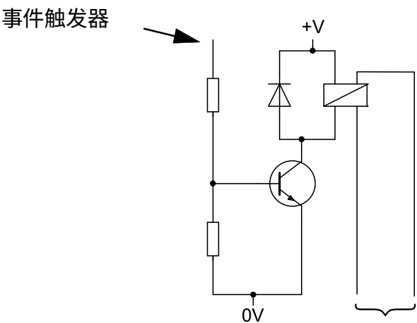
图 8-3：典型继电器电路 - 无电压选项
