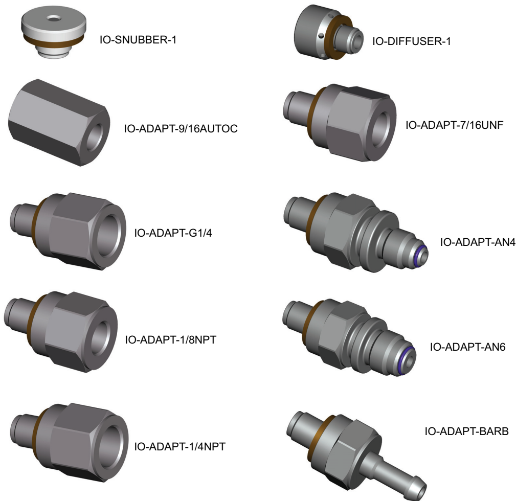
图 2-1：压力适配器
