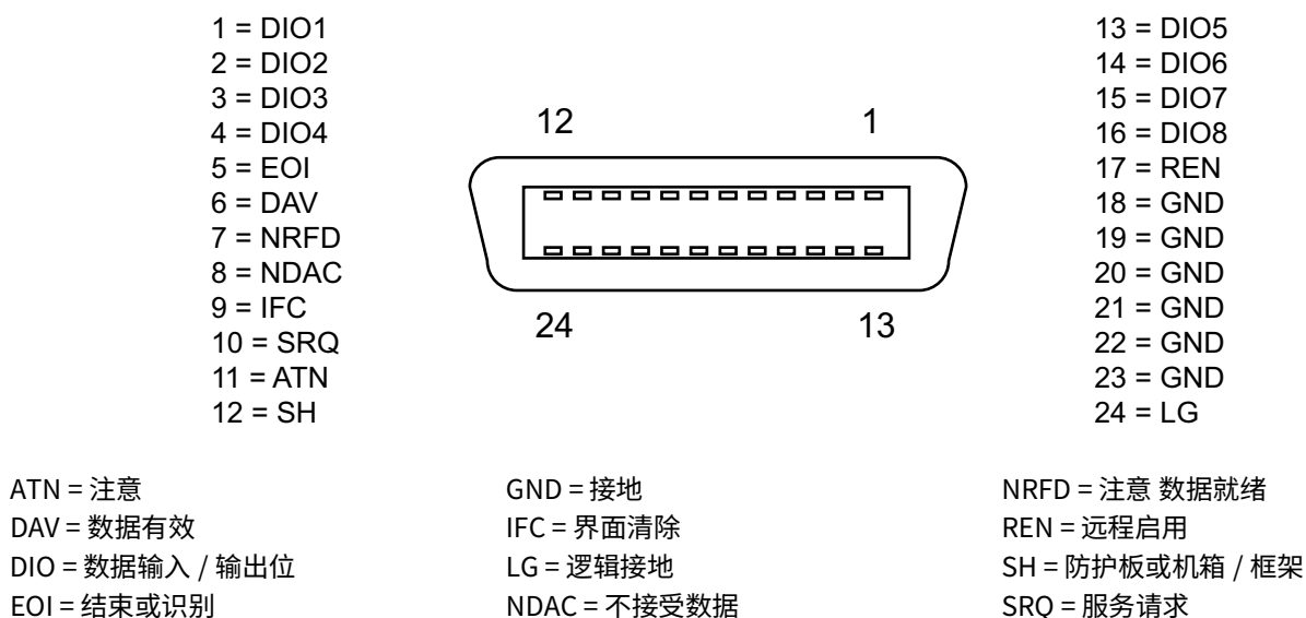
图 2-8: GPIB IEEE 488 连接器引脚排列
