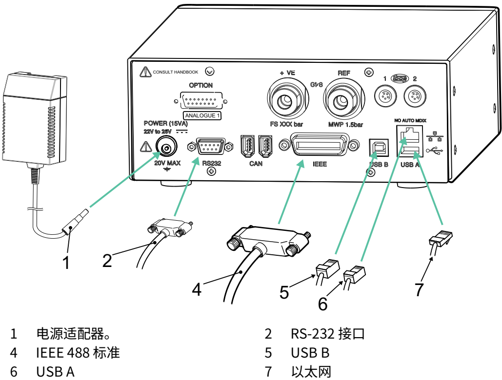
图 2-6：通信连接器
