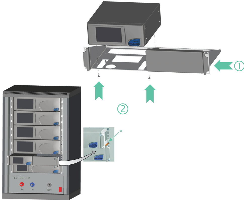
图 2-4：机架安装
