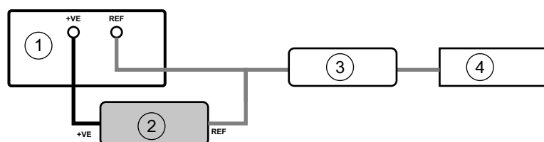
图 7-1：推荐的无管路压力表连接
