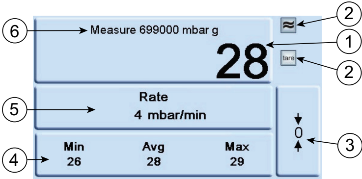
图 3-2：典型测量模式屏幕
